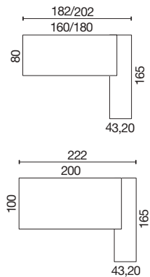
Bureaux sur retour porteur
