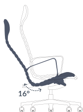
Mécanisme basculant décentré Forward axis tilt mechanism Excentrisch kantelmechanisme
