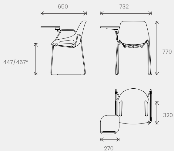
Piètement traineau avec tablette - Sled base with writing shelf - Sledeonderstel met schrijfplateau
